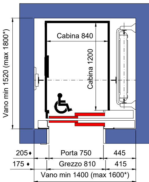
PIANTA VANO CORSA TELAIO PORTE NF (EI120)
