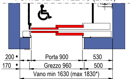
PIANTA VANO CORSA PORTE SENZA TELAIO (E1120)
