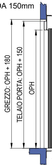
SEZIONE PORTE SENZA TELAI (E1120)
